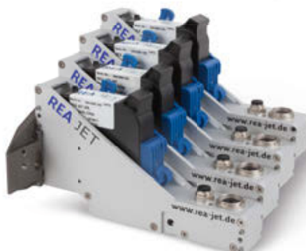
Schreibköpfe
